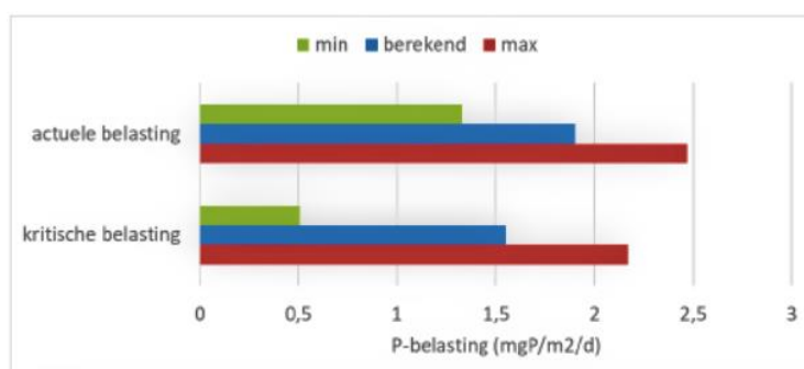
Figuur 5 Actuele en kritische fosfaatbelasting met onzekerheidsmarges 40% voor de kritische belasting en 30% voor de actuele belasting
