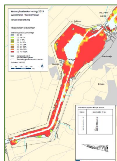
Figuur 21 Totale bedekking waterplanten Wolderwijd en Nuldernaau 2019
