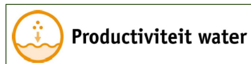
Figuur 4 Sleutelfactor Productiviteit water
