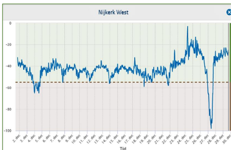
Figuur 16 Waterhoogten december 2020 Nijkerk West
