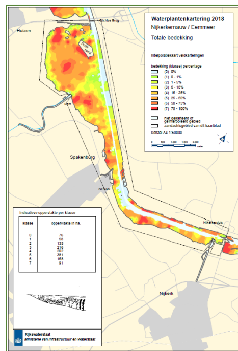
Figuur 22 Totale waterplanten bedekking Eemmeer/Nijkerkernauw 2018
