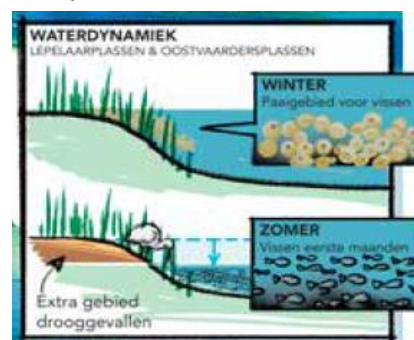
Figuur 19 Groeicyclus vissen bij natuurlijk peilverloop
