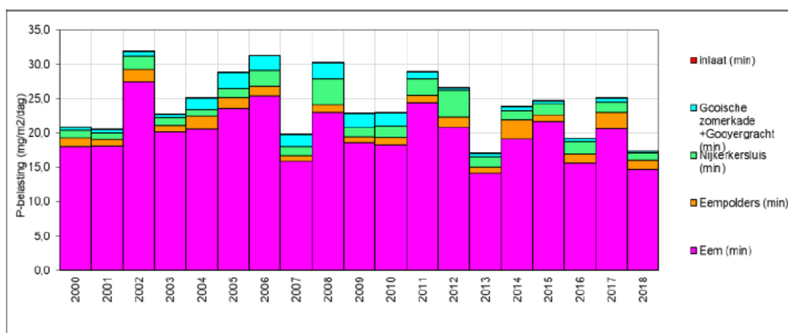
Figuur 10 Berekende fosfaat-belasting (mg/m²/dag) op jaarbasis opgesplitst per bron voor het Eemmeer
