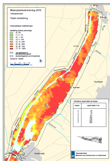
Figuur 20 Totale waterplanten bedekking Veluwemeer 2019
