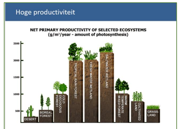
Figuur 12 Organische productie in diverse ecosystemen
